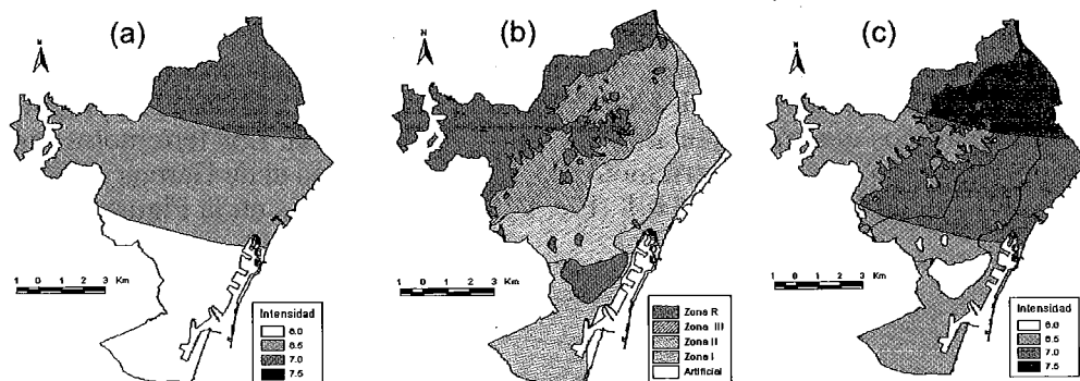
Figura 2. (a) Mapa de peligrosidad determinista para suelo medio en términos de intensidad; (b) Zonación sísmica basada en efectos locales (Cid et al., 2001); (c) Mapa de peligrosidad determinista con efectos locales en términos de intensidad.
