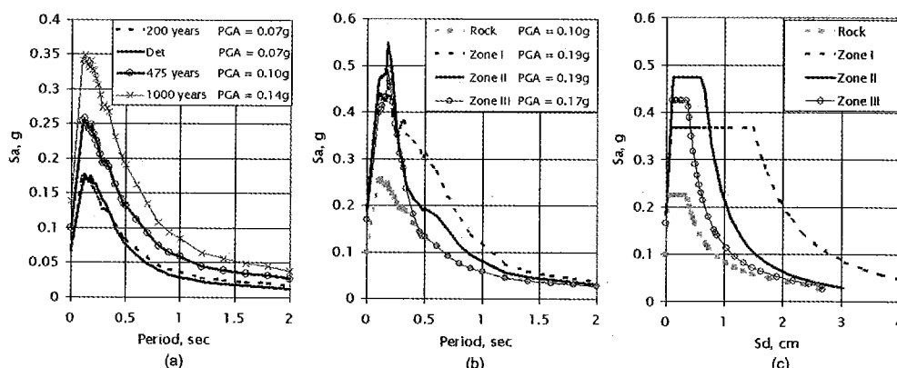
Figura 3. (a) Espectros de respuesta de aceleración probabilistas y determinista para un suelo medio en Barcelona; (b) Espectros de respuesta de aceleración probabilista para las diferentes zonas de suelo y un período de retorno de 475 años; (c) Formas analíticas de los espectros de demanda para las diferentes zonas de suelo y un período de retorno de 475 años.
