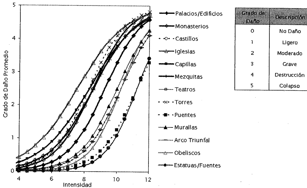
Figura 4. Curvas de Vulnerabilidad promedio para las tipologías de monumentos y su descripción de daños.
