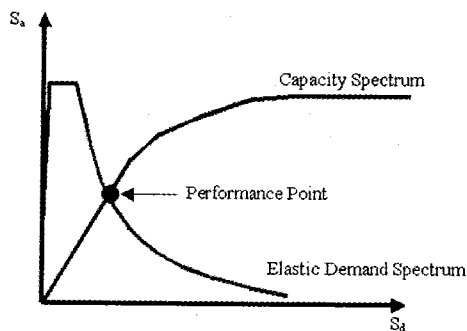
Figura 5. Diagrama del método del espectro de capacidad.
