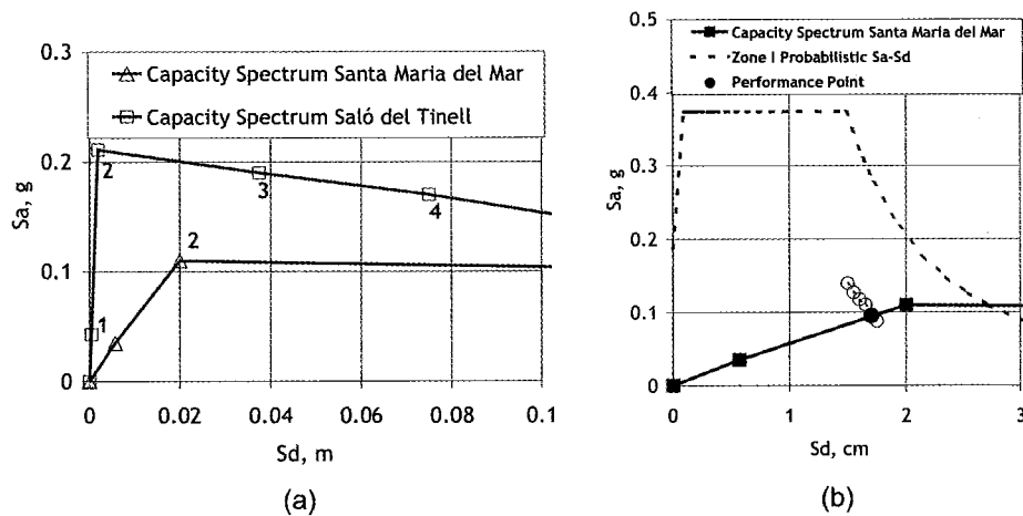
Figura 9. (a) Curvas de capacidad obtenidas para la iglesia de Santa María del Mar y el Salón del Tinell; (b) Punto de desempeño para la iglesia de Santa María del Mar en el escenario probabilista.
