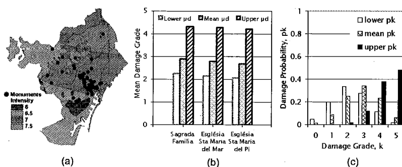
Figura 7. (a) Peligrosidad determinista que afecta a los monumentos analizados; (b) Los 3 monumentos con el mayor grado de daño para el escenario determinista; (c) Distribución de la probabilidad de daño para la Iglesia de Sagrada Familia para el escenario determinista.
