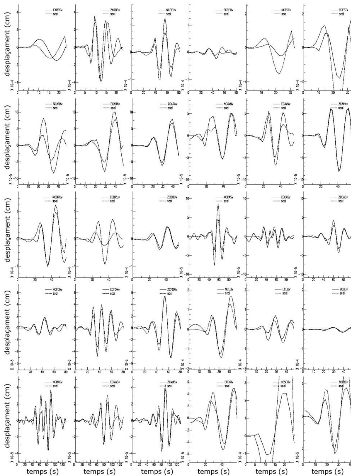
Figura 4. Formes d'ona de les estacions de la xarxa sísmica de Catalunya corresponents al sísmes ocorregut el dia 3 d'abril de 2019 a les 15:29:51 (TU), amb epicentre a l'Alt Urgell, juntament amb les formes d'ona teòriques (scal).
