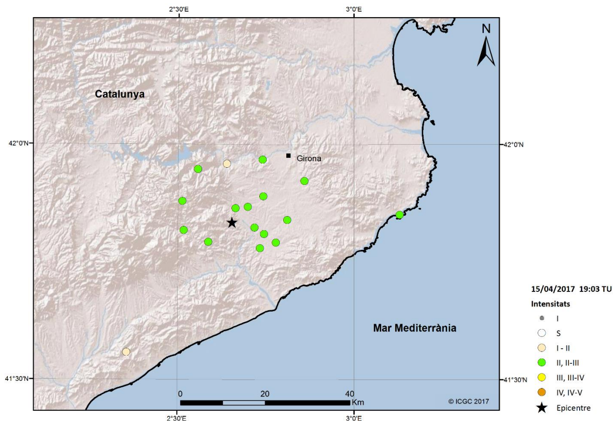
Figura 11. Mapa d'intensitats corresponent al sisme del dia 15/04/2017 a les 19:03 (TU).
