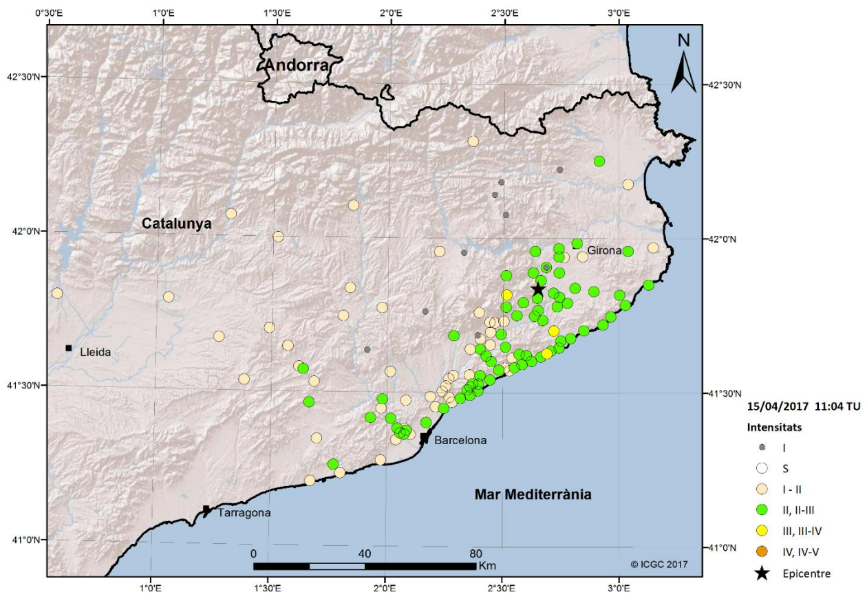
Figura 10. Mapa d'intensitats corresponent al sisme del dia 15/04/2017 a les 11:04 (TU).
