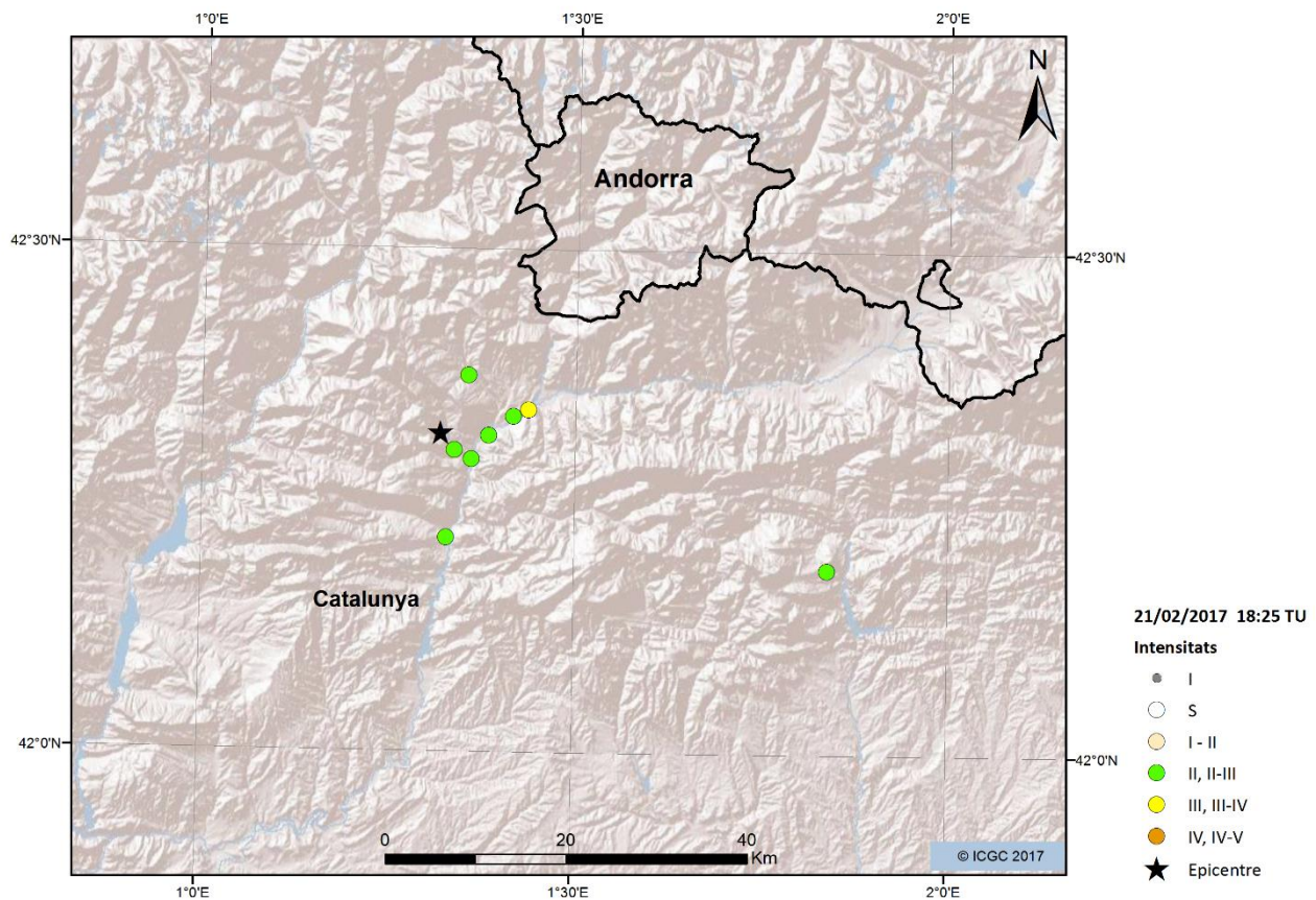
Figura 8. Mapa d'intensitats corresponent al sisme del dia 21/02/2017 a les 18:25 (TU).
