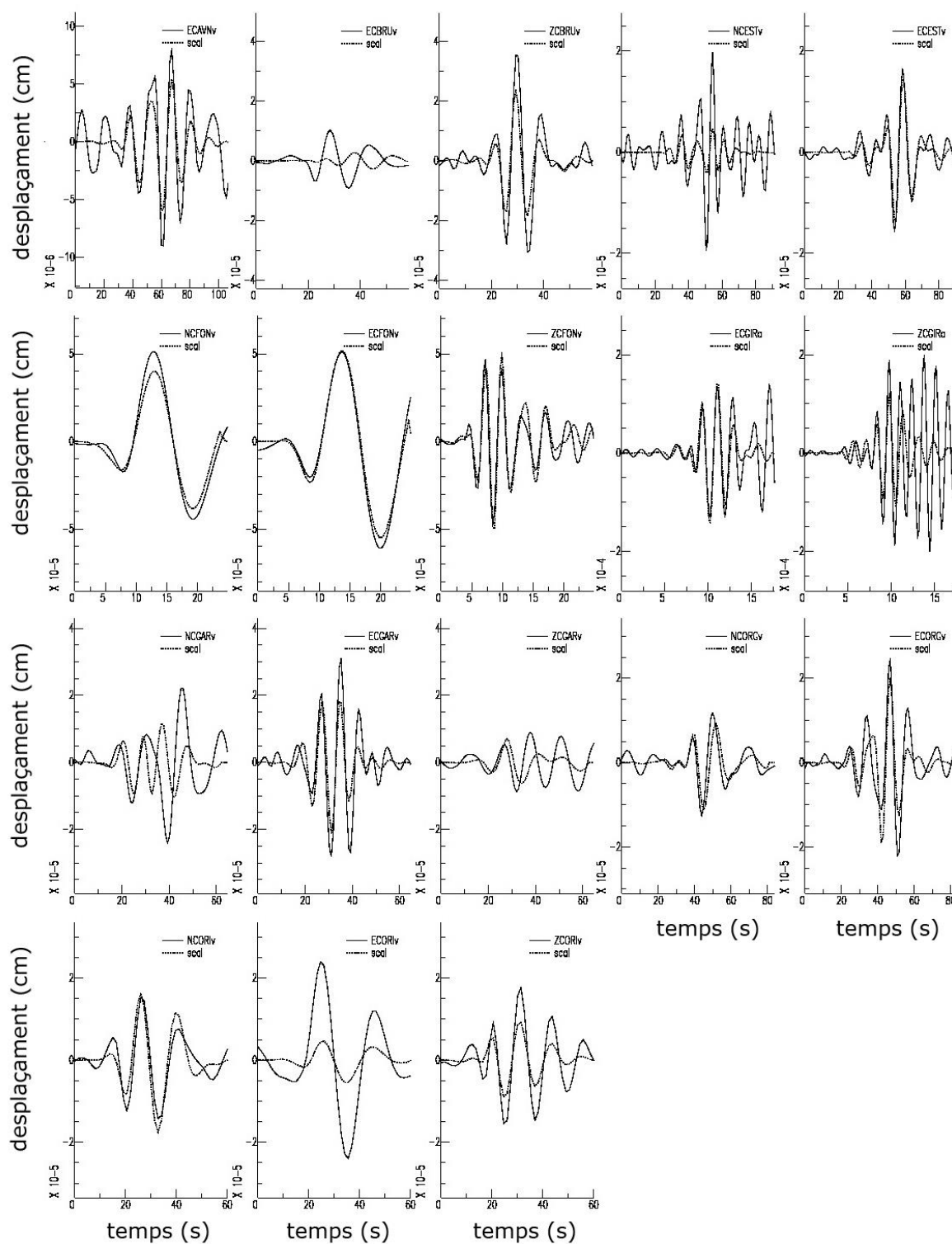
Figura 4. Formes d'ona de les estacions de la xarxa sísmica de Catalunya corresponents al sisme ocorregut el dia 5 d'abril de 2017 a les 11:04:36 (TU) amb epicentre a la Selva, junt amb les formes d'ona teòriques (scal).
