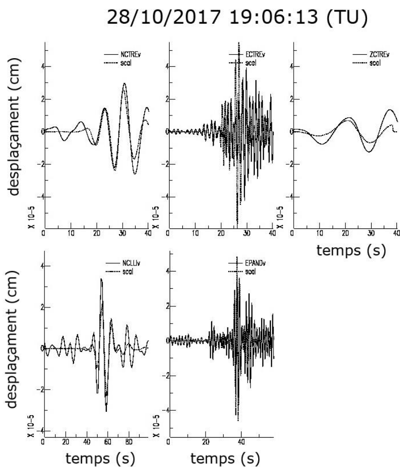
Figura 6. Formes d'ona de les estacions de la xarxa sísmica de Catalunya corresponents al sisme ocorregut el dia 28 d'octubre de 2017 a les 19:06:13 (TU), amb epicentre als Hautes-Pyrénées, junt amb les formes d'ona teòriques (cal).
