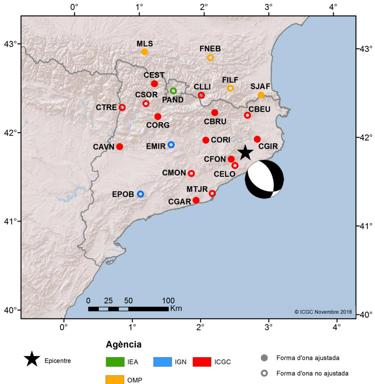
Figura 3. Localització epicentral del sisme ocorregut el dia 15 d'abril de 2017 a les 11:04:36 (TU), amb epicentre a la Selva, representada per una estrella; situació de les estacions sísmiques les dades de les quals s'han utilitzat per a calcular el mecanisme focal d'aquest sisme: els cercles plens mostren les estacions proveïdores de dades que s'han pogut ajustar al càlcul i els cercles buits les que no s'han pogut ajustar. També es mostra el mecanisme focal resultant del càlcul.
