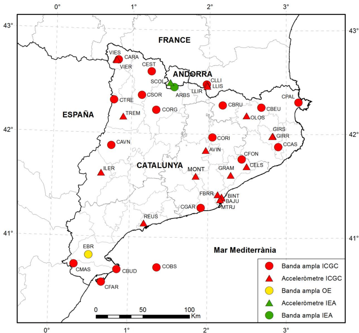
Figura 1. Situació de les estacions sísmiques de la xarxa sísmica de Catalunya el 2016, a Catalunya i Andorra. S'indiquen, amb diferents símbols, els diferents tipus d'estació. El sismòmetre ARBS i l'acceleròmetre SCOL, instal·lats a Andorra, són fruit d'una col·laboració entre l'Institut d'Estudis Andorrans (IEA) i l'ICGC.
