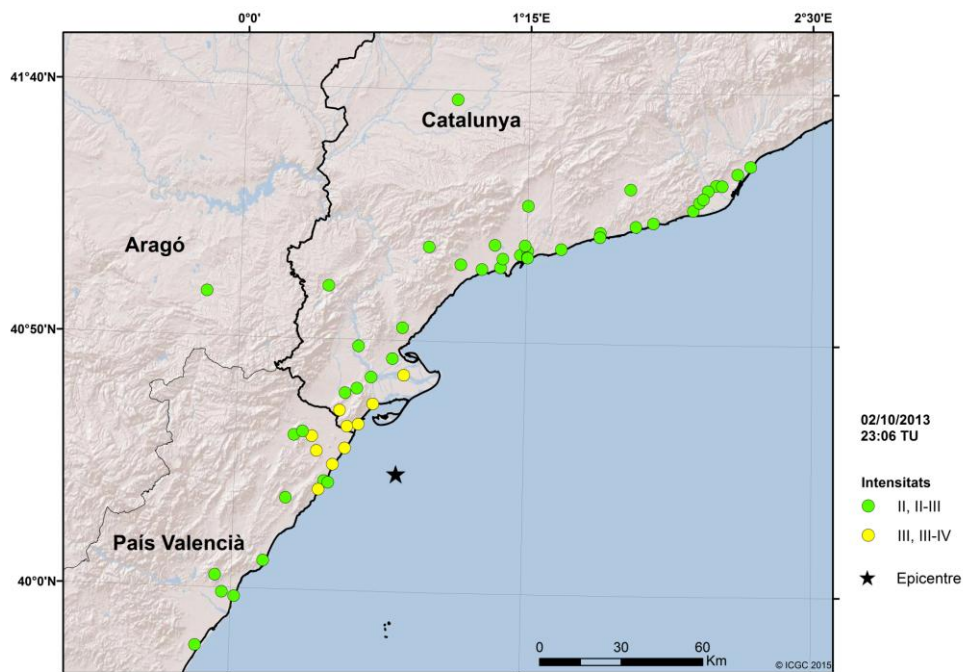
Figura 6. Mapa d'intensitats corresponent al sisme del dia 2/10/2013 a les 23:06 (TU).
