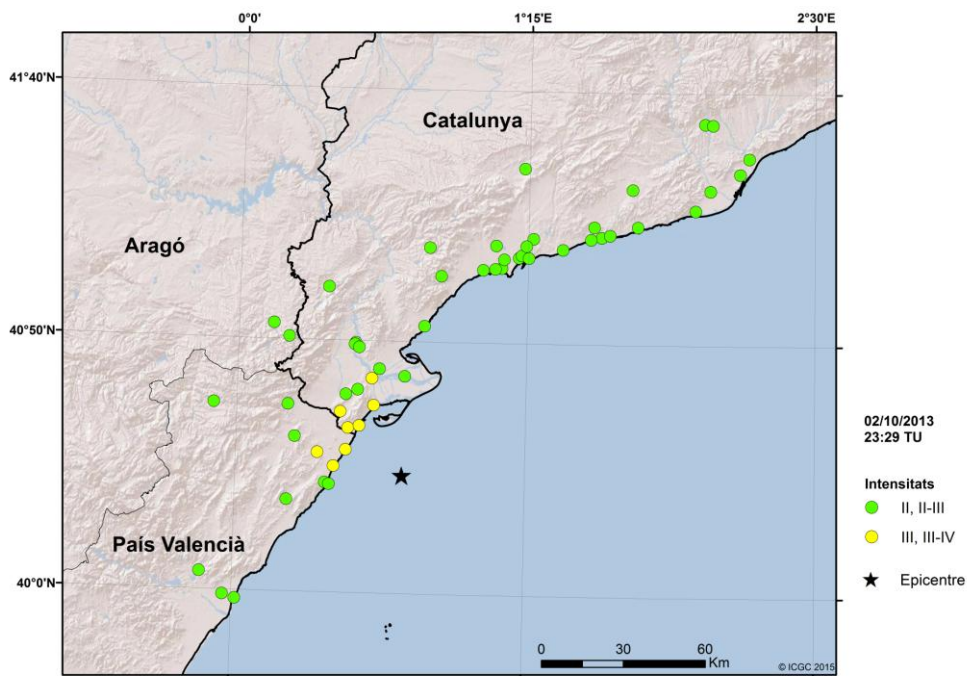
Figura 7. Mapa d'intensitats corresponent al sisme del dia 2/10/2013 a les 23:29 (TU).
