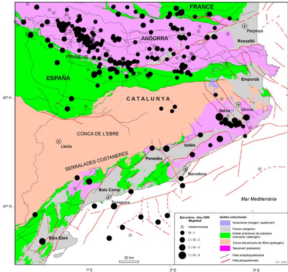
Figura 8. Sismicitat de l'any 2008 en el context estructural de Catalunya (SGC, 1991) extret del Mapa geològic de Catalunya a escala 1:250 000 (SGC, 1989). Es representen els epicentres sobre les principals unitats estructurals i les falles -que inclouen els encavalcaments- diferenciades segons l'edat de la seva activitat tectònica (anteplioquaternària, més de 6 milions d'anys i plioquaternària, menys de 6 milions d'anys).
