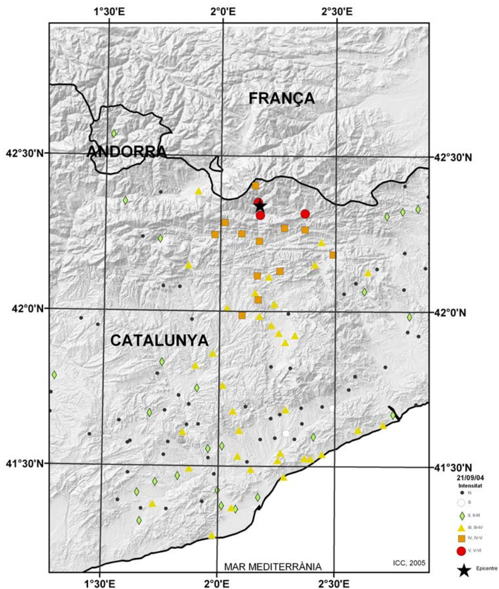
Figura 6. Distribució d'intensitats del sisme de 21 de setembre de 2004. La situació de l'epicentre es representa mitjançant l'estel.
