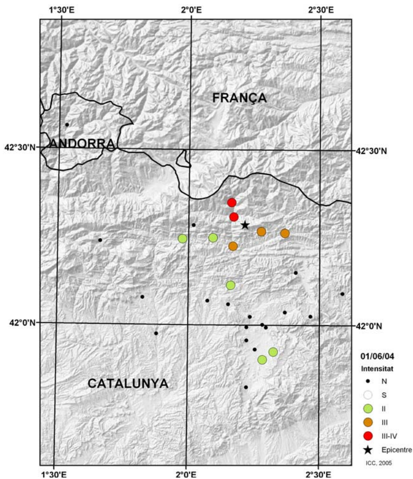
Figura 5. Distribució d'intensitats del sisme de 1 de juny de 2004. La situació de l'epicentre es representa mitjançant l'estel.
