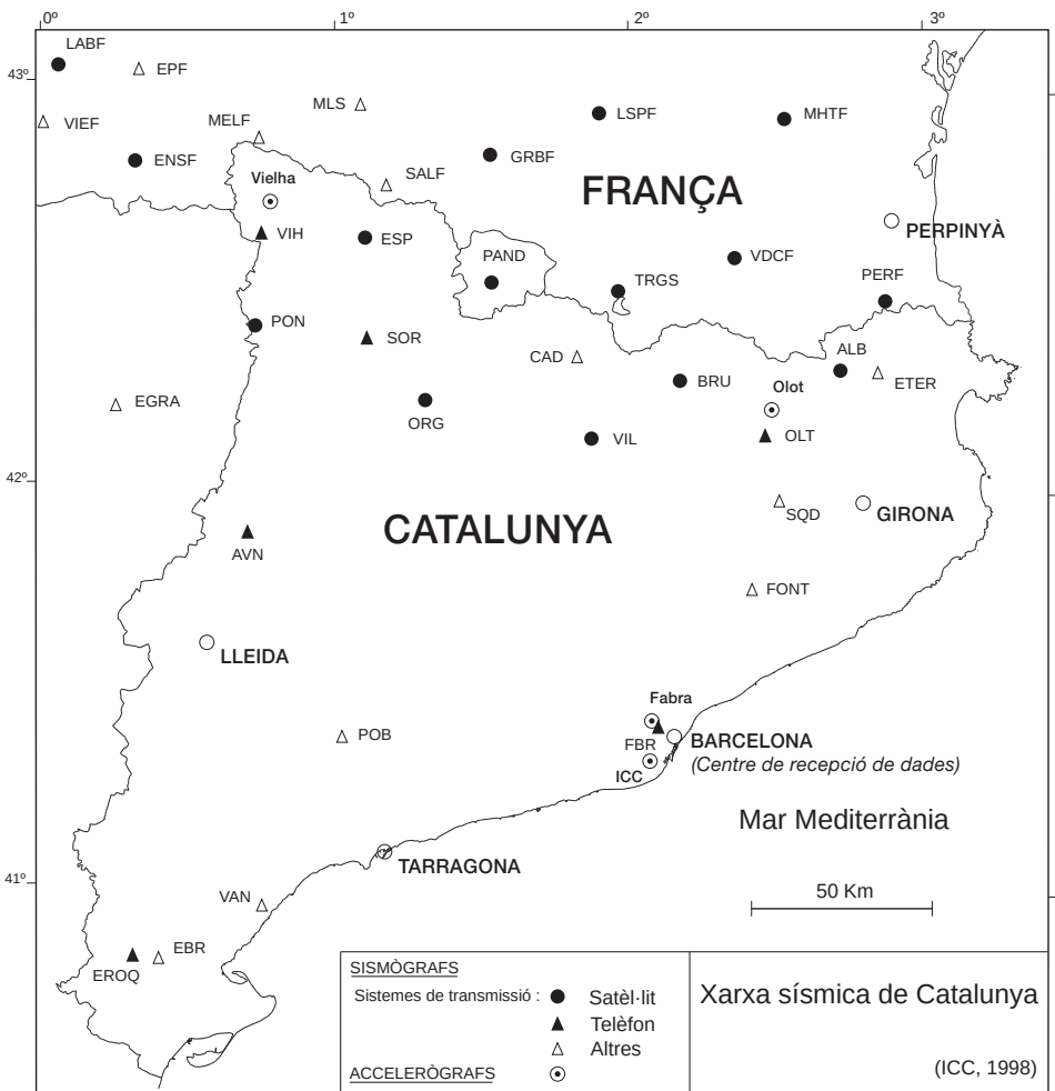
Figura 1. Situació de les estacions sísmiques a Catalunya i regions veïnes (1997). S'indica, amb diferents símbols, els diferents tipus d'equipaments.
