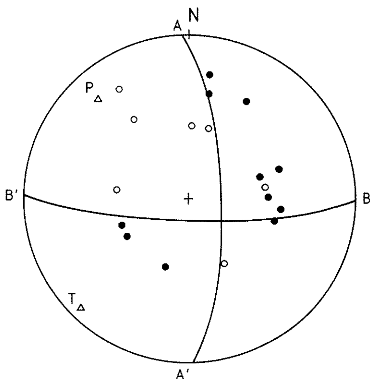
Figura 5. Mecanisme focal: rodones plenes indiquen compressió i buides dilatació. Projectió de la semiesfera inferior. Es donen també l'azimut i el cabussament dels plans nodals i dels eixos de pressió i tensió.
