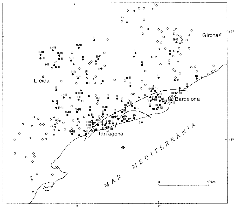
Fig. 4: Mapa d'isosistes corresponent al terratrèmol 24/08/87. L'asterisc representa la localització instrumental.
