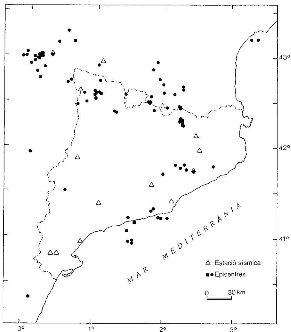
Fig. 6: Situació de les determinacions epicentrals dels sismes corresponents a l'any 1987. Els quadrats representen localitzacions gràfiques i els cercles localitzacions amb ordinador
