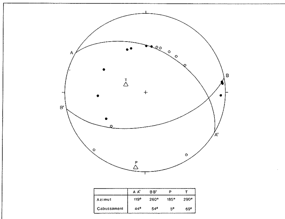
Fig. 5: Mecanisme focal: rodones plenes indiquen compressió i buides dilatació. Projectió de la semiesfera interior. Es donen també l'azimut i el cabussament dels plans nodals i dels eixos de pressió i tensió.
